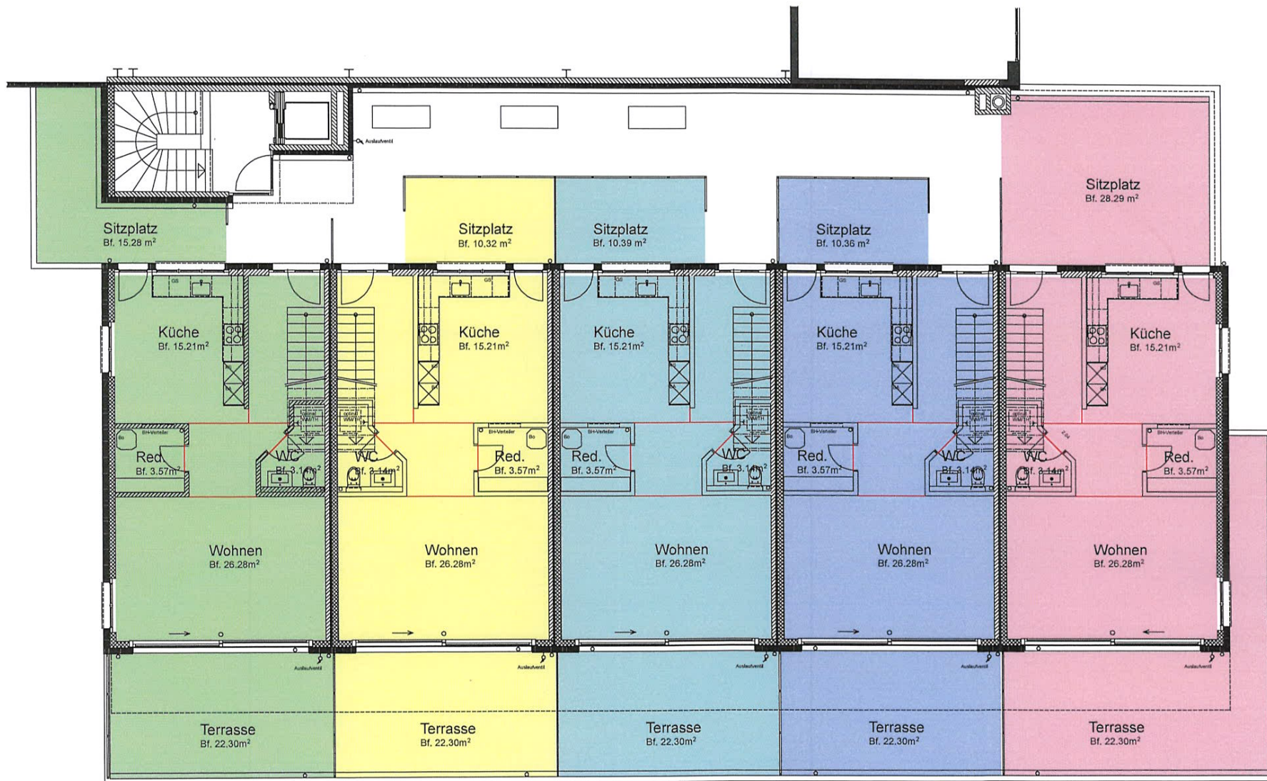
Obergeschoss M. 1:100
